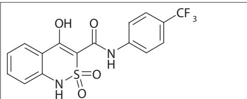
Рисунок. Хімічна формула N -(4-трифлуорометилфеніл)-4-гідрокси-2,2-діоксо-1 H -2λ 6 ,1-бензотіазин-3-карбоксаміду
